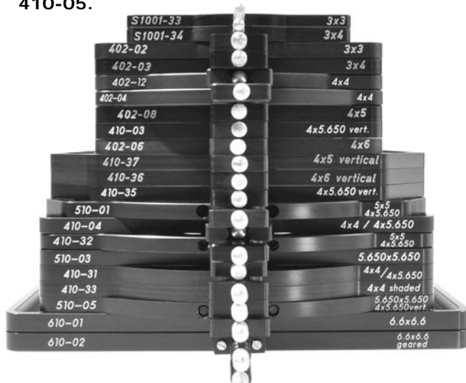
Filterhalter 410-38 für Rundfilter in einer 150mm Bühne.
